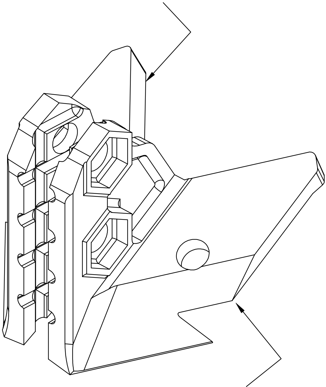
KAG 008 - LH Mulch Blade Adapter
