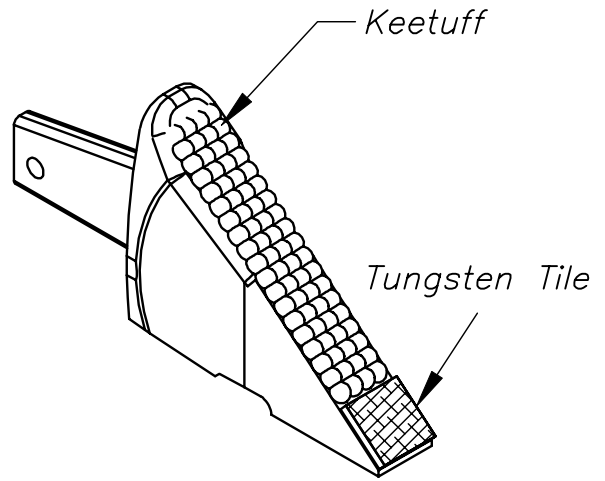
DDP18WT
