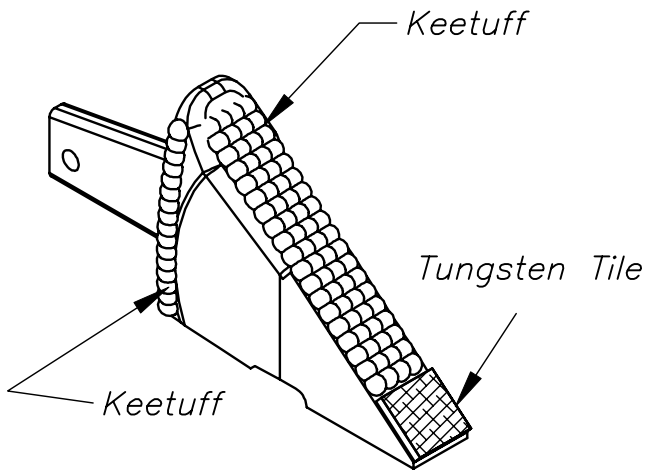
DDP18WT1
